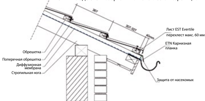
СХЕМА ВОДОСТОКА. Вариант 1-ый с нахлестом черепицы.
